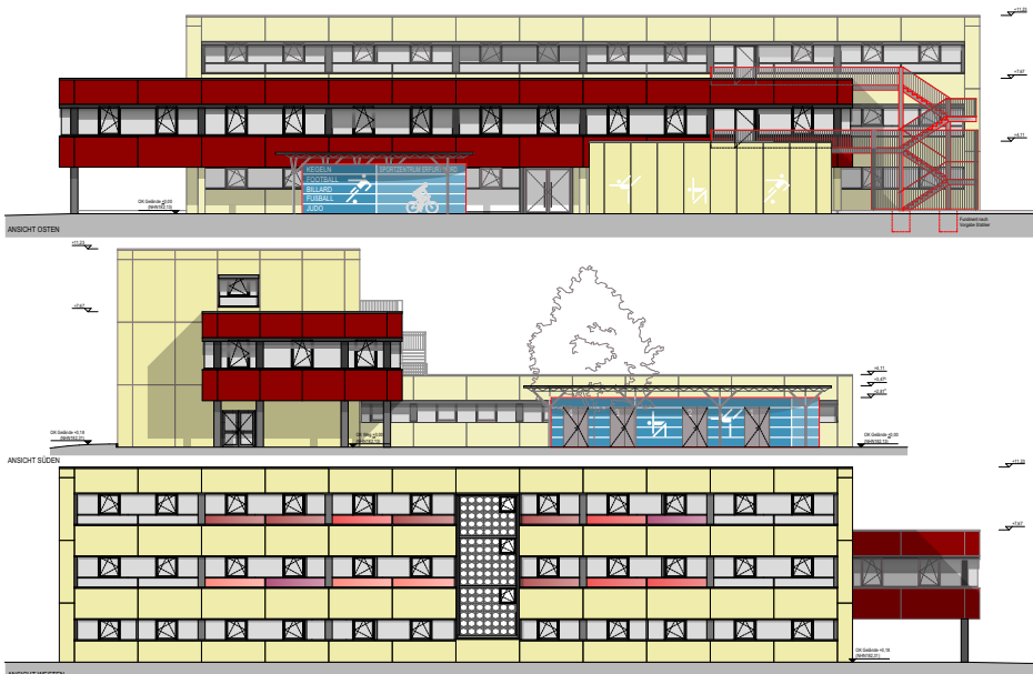
Pläne zur Neugestaltung des Sportkomplexes Rieth in der Essener Straße, Erfurt
